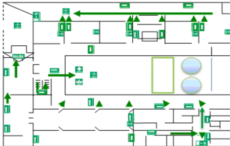
Plano o croquis del equipo de contra incendios
